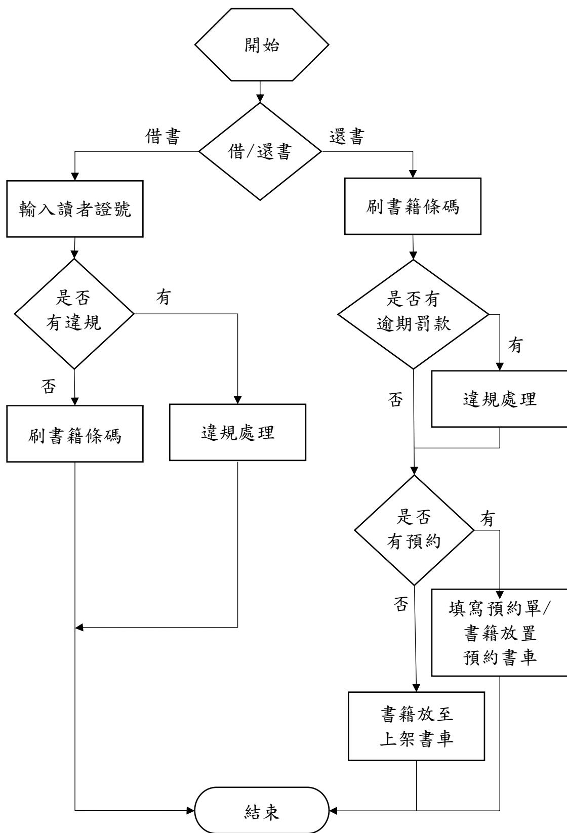
圖62：借還書服務
