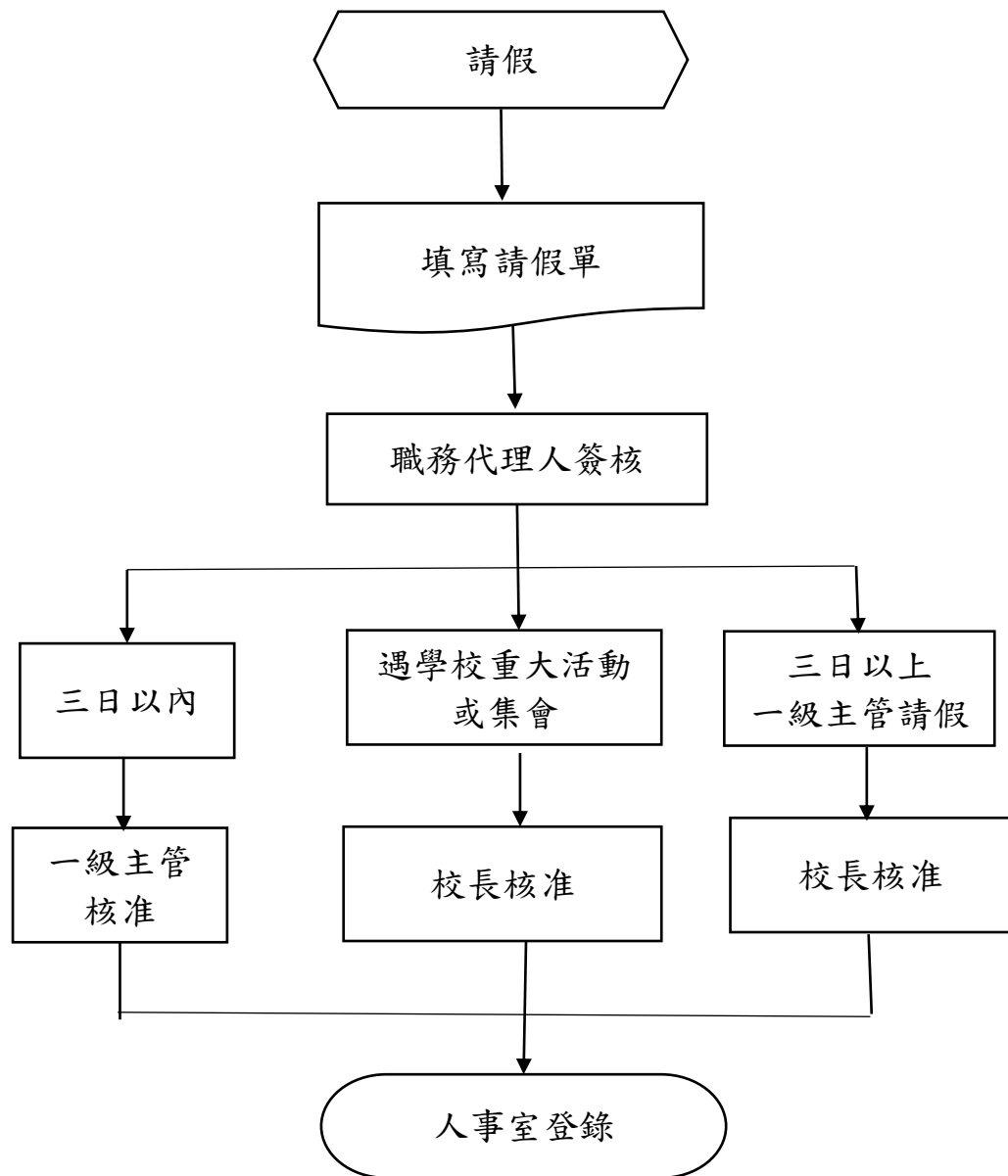
圖10：請假作業
