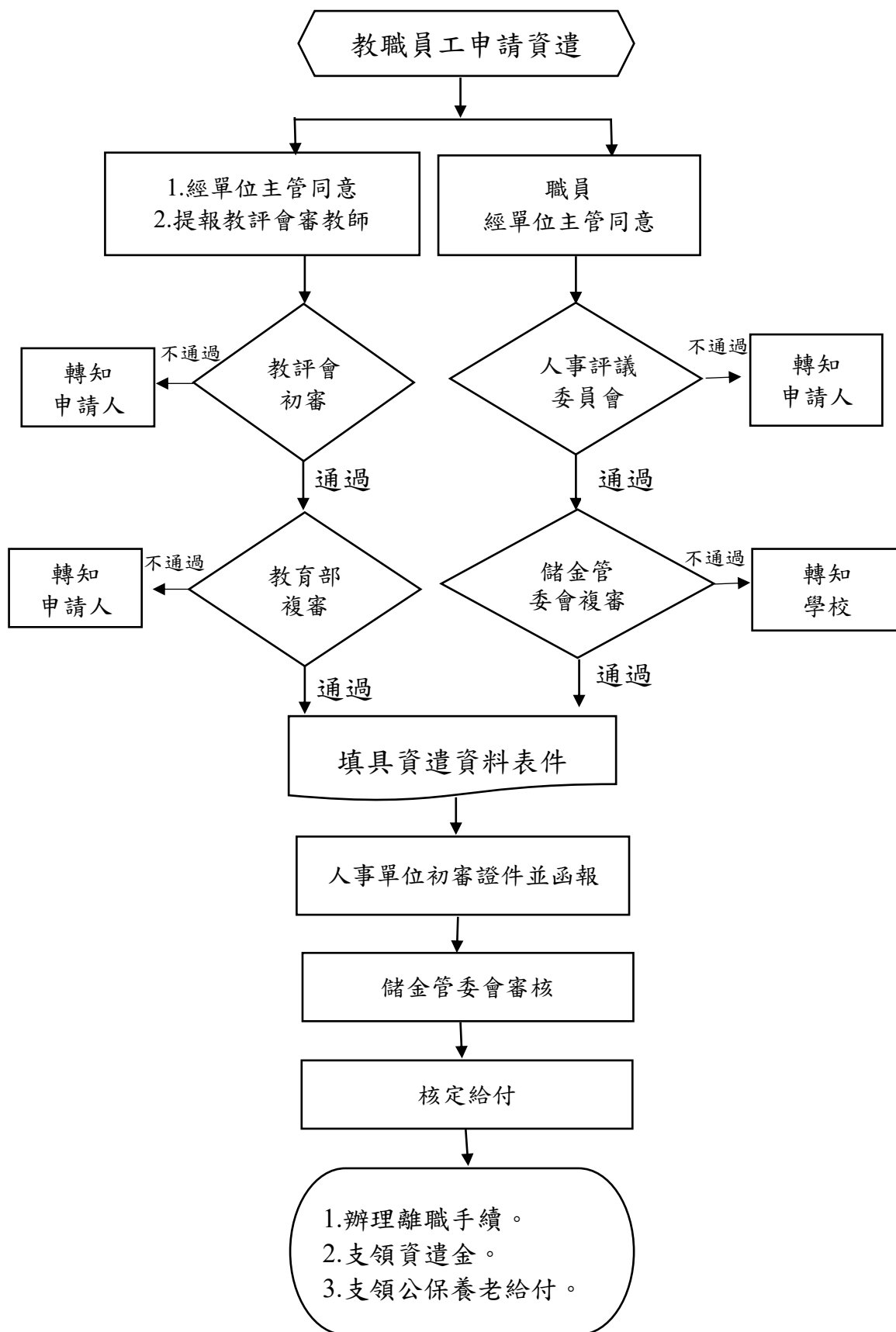
圖9：資遣作業
