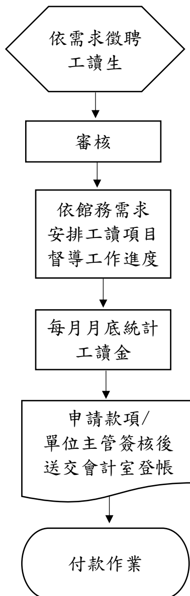
圖59：工讀生管理
