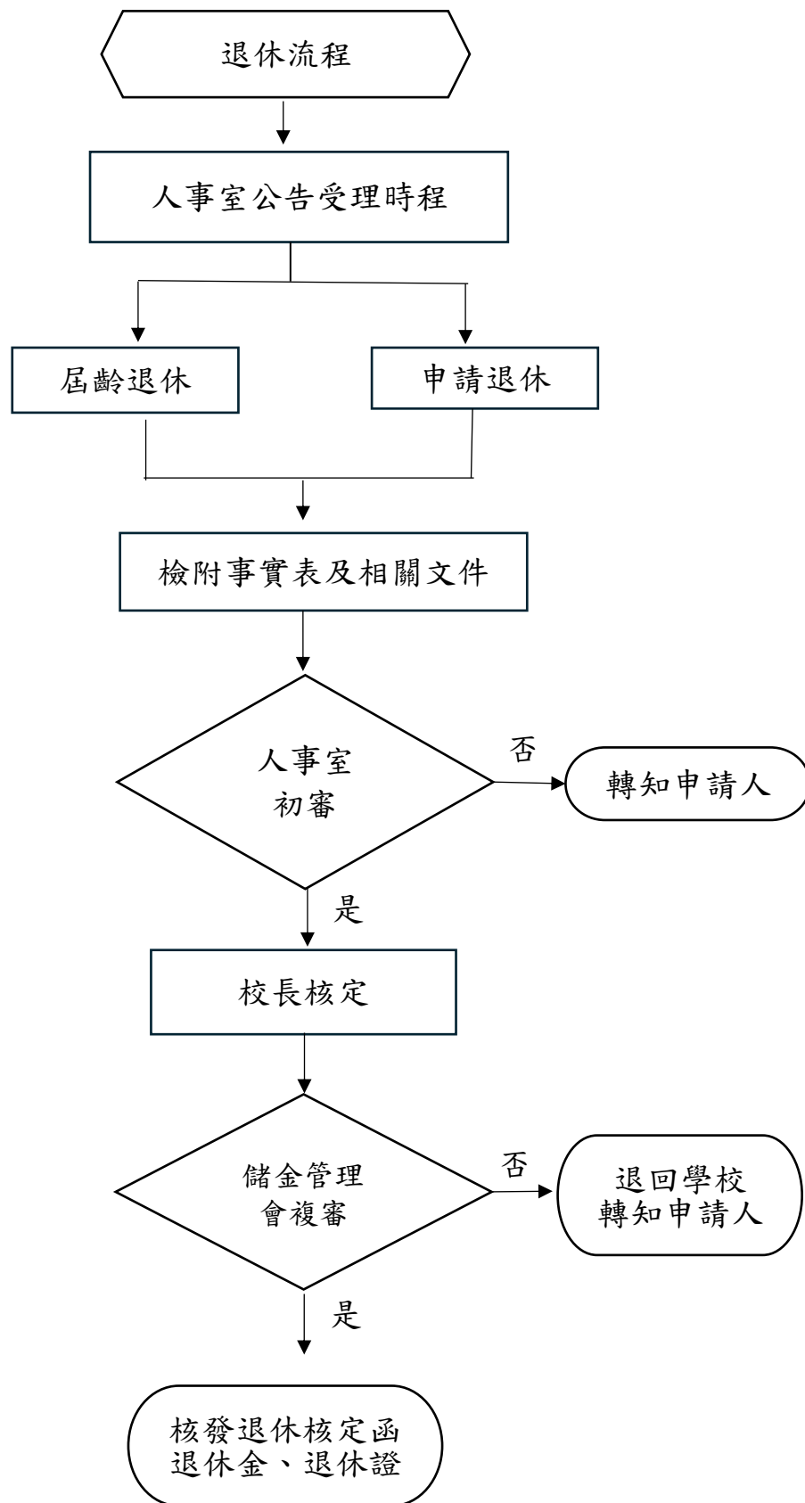
圖7：退休作業
